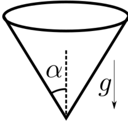
Рис. 2: Конус в поле тяжести
