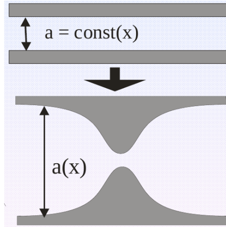
Рис. 1: Адиабатический квантовый транспорт
