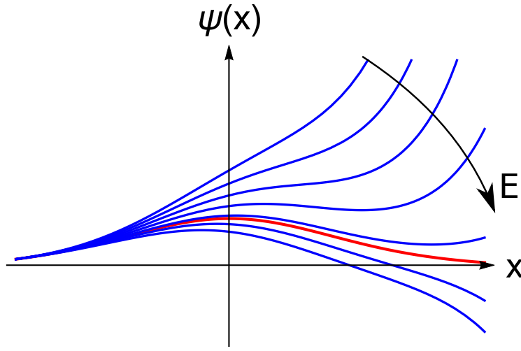
Рис. 1: Поведение волновой функции при различных энергиях
