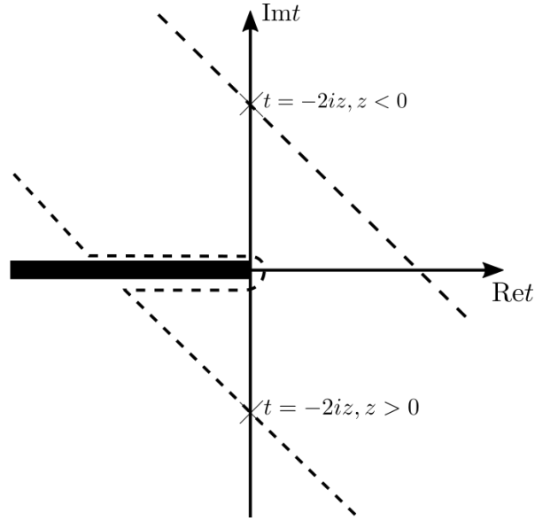
Рис. 4.3: Структура комплексной плоскости и контур интегрирования для задачи Ландау-Зенера
