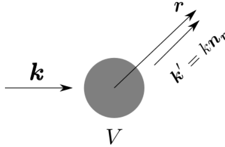
Рис. 8.1: Задача рассеяния в многомерном пространстве.
