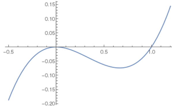
Рис. 11.4: Перевёрнутый потенциал -U(x) . Оси в единицах \eta ( Ox ) и \omega ( Oy ).
