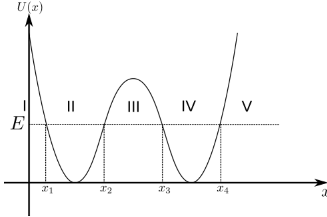
Рис. 7.4: Двухъямный потенциал
